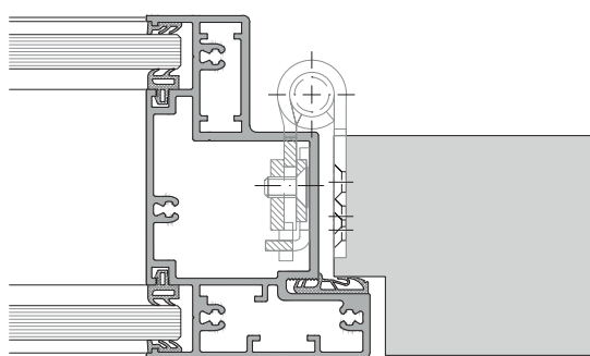
Door element hinge side
